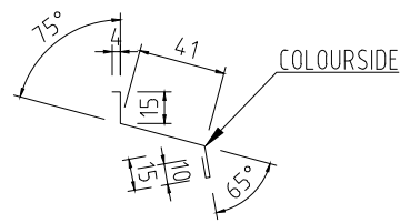
UNDERBLECK FÖNSTER 40 Tj=0,6 L=1200, 1500, 2000mm KB=85mm
