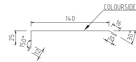
GAVELBESLAG RAK 25x140 Tj=0,5-0,6 L=2000mm KB=213mm
