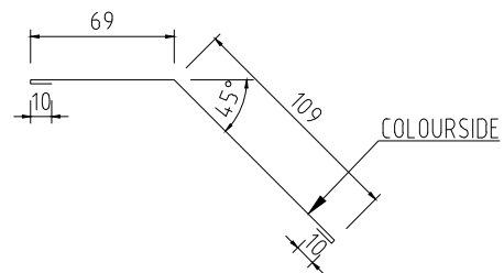
FOTPLÅT 69x109 VÄNDBAR Tj=0,5-0,6 L=2000mm KB=198mm
