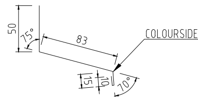
ÖVERBLECK FÖNSTER 80 Tj=0,6 L=1200, 1500, 2000mm KB=158mm
