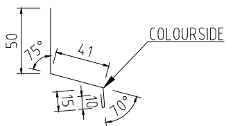
ÖVERBLECK FÖNSTER 40 Tj=0,6 L=1200, 1500, 2000mm KB=116mm
