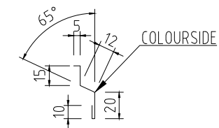
TRÖSKELBLECK 1230 Tj=0,5-0,6 L=1230mm KB=62mm
