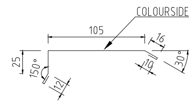
GAVELBESLAG RAK 25x105 Tj=0,5-0,6 L=2000mm KB=178mm
