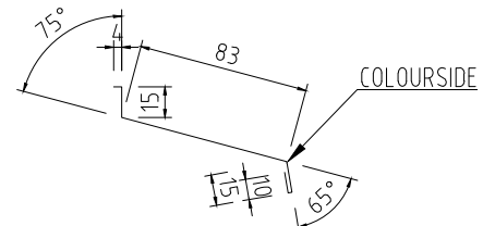
UNDERBLECK FÖNSTER 80 Tj=0,6 L=1200, 1500, 2000mm KB=127mm
