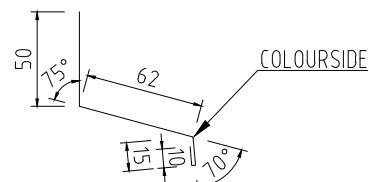
ÖVERBLECK FÖNSTER 60 Tj=0,6 L=1200, 1500, 2000mm KB=137mm
