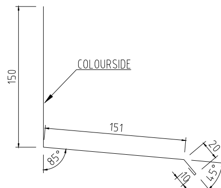
STÄNSKIVA 170x150 Tj=0,5-0,6 L=2000mm KB=331mm
