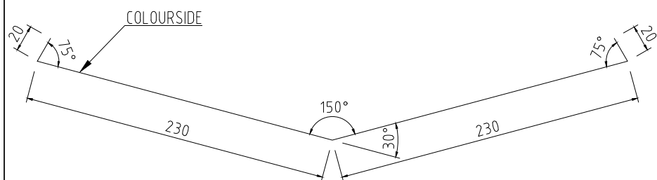
RÄNNDALSPLÅT RAK 230x230 Tj=0,5-0,6 L=2000mm KB=500mm
