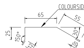
GAVELBESLAG KNÄCKT 25x65x55 Tj=0,5-0,6 L=2000mm KB=177mm
