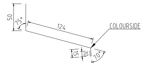
ÖVERBLECK FÖNSTER 120 Tj=0,6 L=1200, 1500, 2000mm KB=199mm
